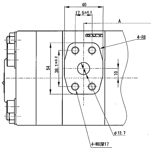
X 矢視図 VIEW OF X
