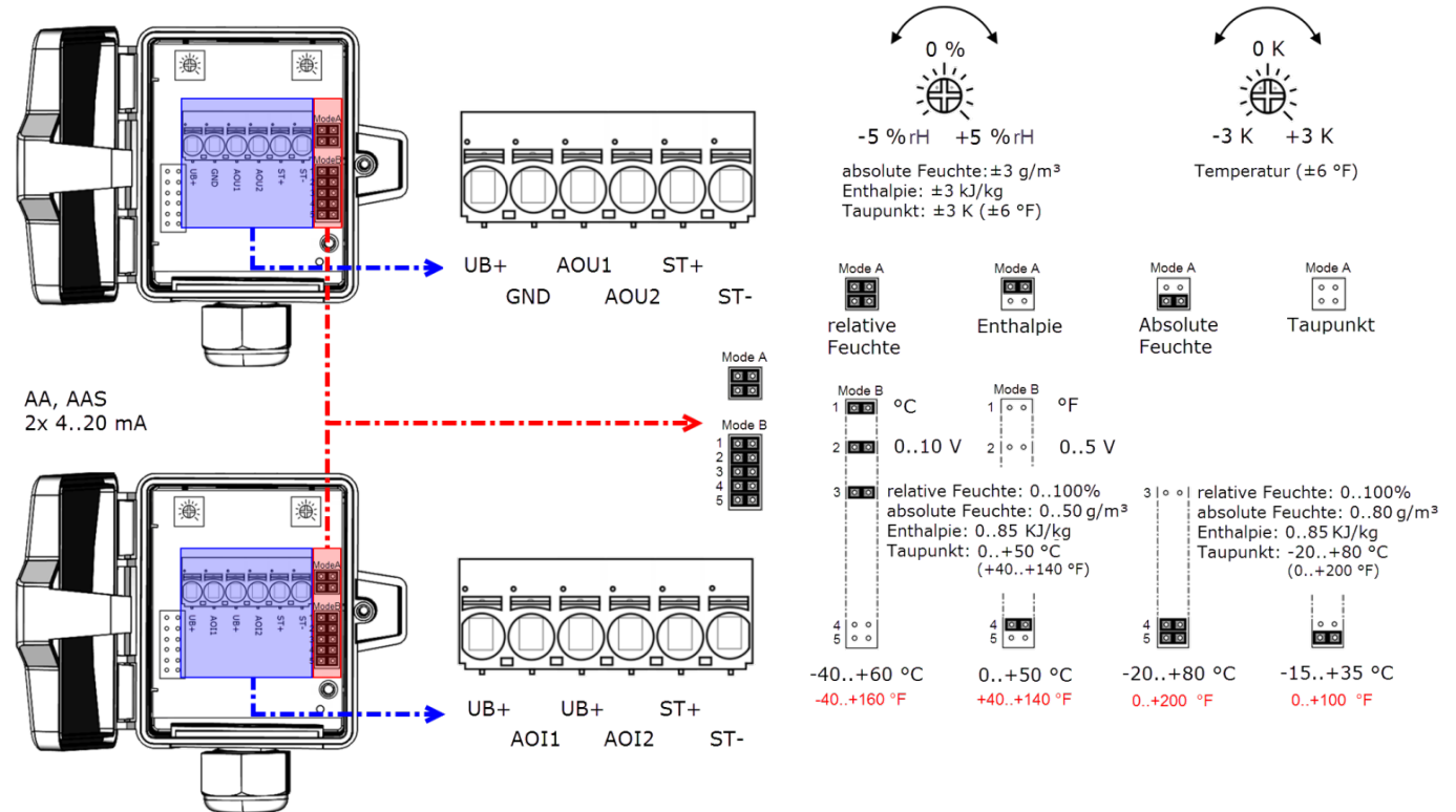
Abb.: (Messbereichs- und Offseteinstellung, Standardeinstellung: -20 °C..+80 °C | 0 K)
